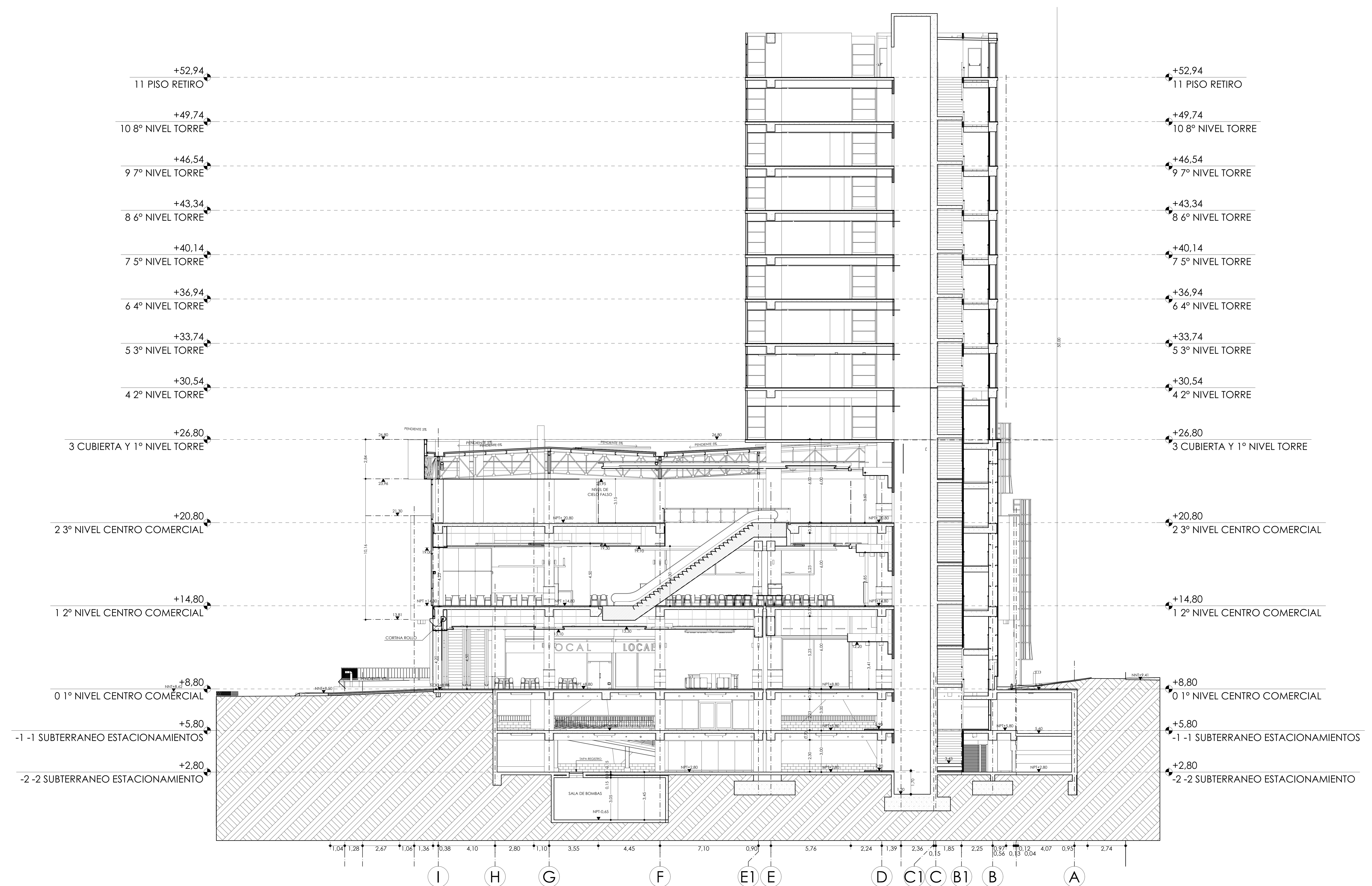
CORTE B-B
